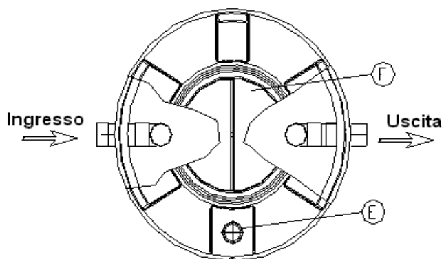
PIANTA
